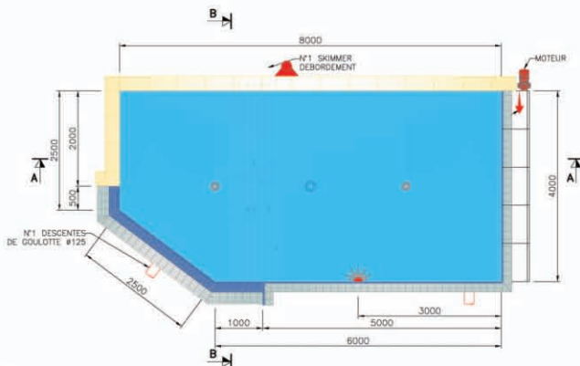
PISCINE FINIE ECHELLE 1:50
