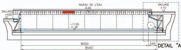
PISCINE FINIE ECHELLE 1:50
